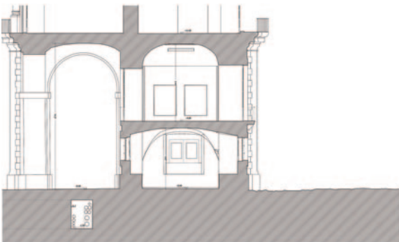
39-42_Sala Sol Lewitt: sezioni verticali vettorializzate e relativo riferimento planimetrico.
