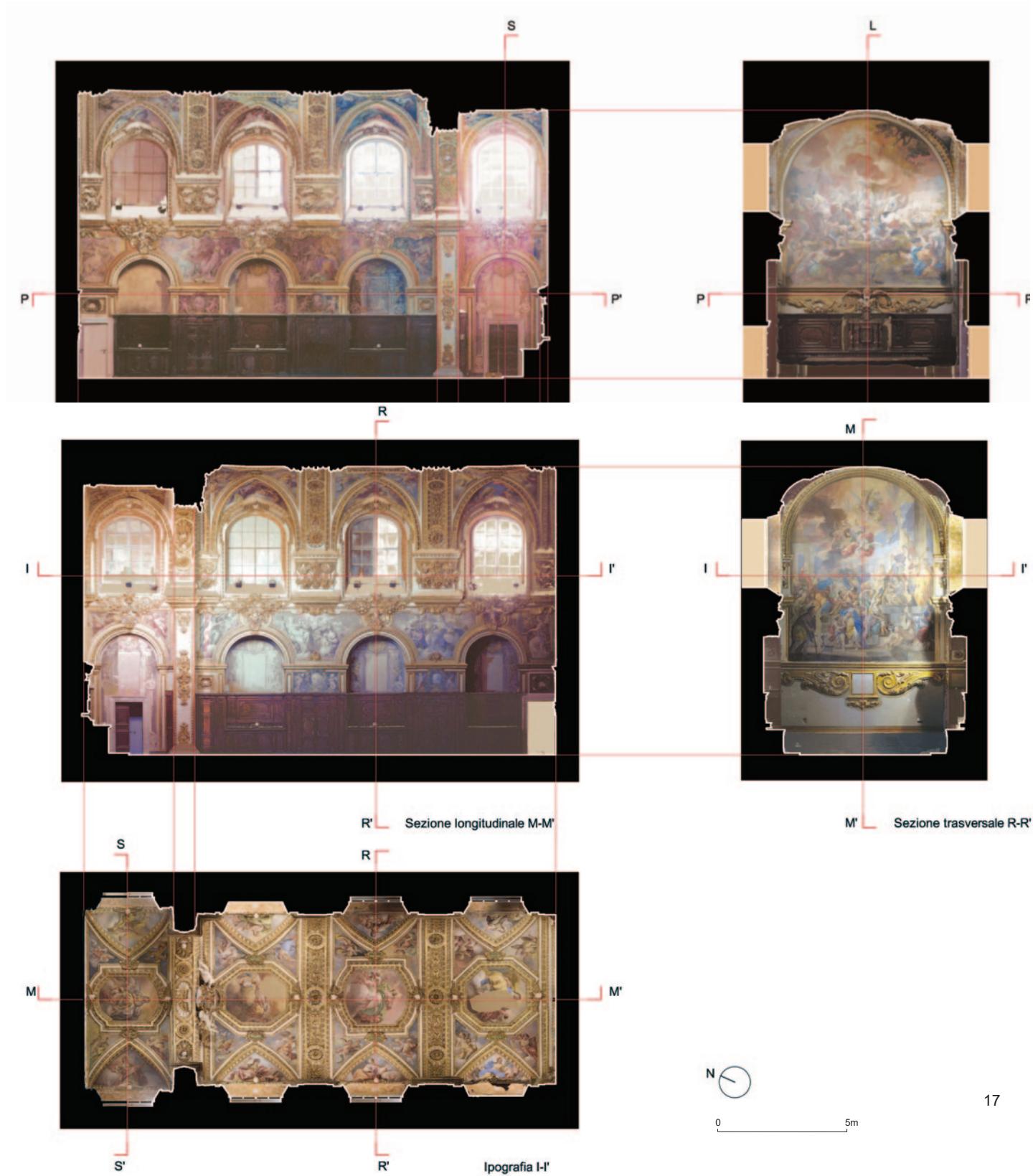
17_Ortoproiezioni in ipografia ed alzato da nuvola dei punti range-based (TLS).
