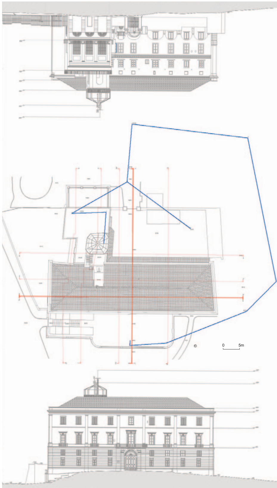
12_Disegni vettorializzati: pianta delle coperture, prospetto nord-est e prospetto principale a sud-ovest.
