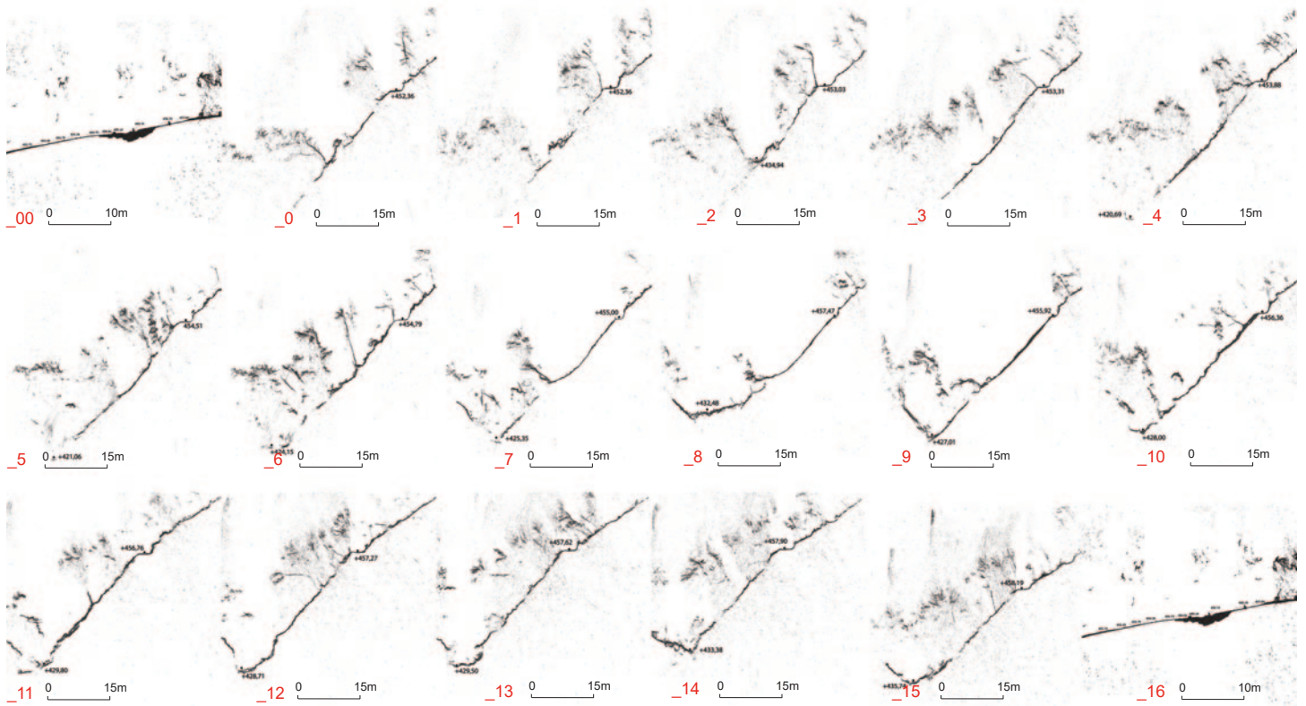
4_Ortoproiezione da nuvola di punti image-based (SAPR). 5_Sezioni trasversali da rilievo integrato (TLS e SAPR).
