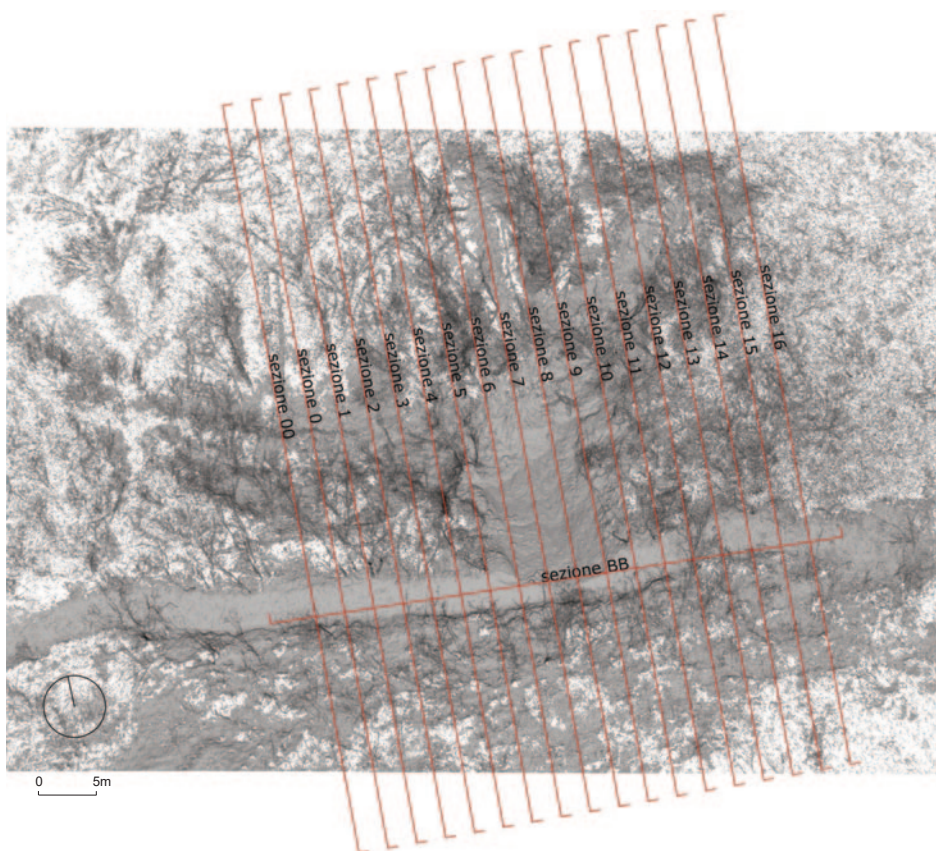
1_Ortoproiezione da nuvola di punti image-based (SAPR). 2_Ortoproiezione da nuvola di punti range-based (TLS). 3_Riferimento planimetrico delle 18 sezioni trasversali, passo 2.5 mt.
