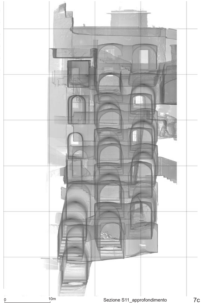
Sezione S11_approfondimento
