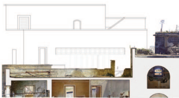
Sezione F-F'
