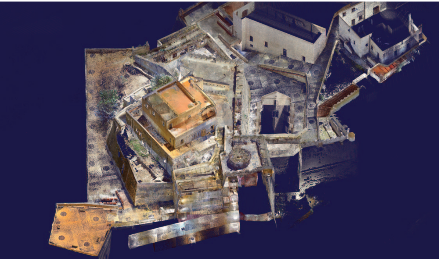
4_Ortoproiezione in alzato da nuvola dei punti image-based (SAPR). 5_Ortoproiezione delle coperture da nuvola dei punti image-based (SAPR). 6_Vista assonometrica da nuvola dei punti range-based (TLS).
