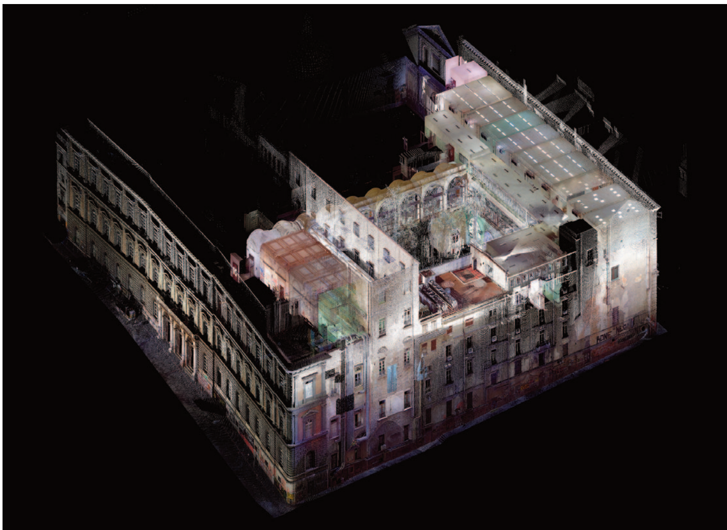
6-8_Viste assometriche della nuvola dei punti range-based (TLS).
